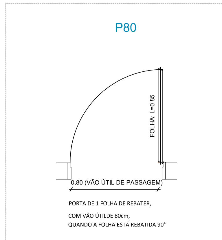
DETALHE PORTA
